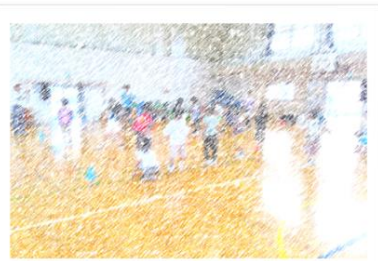
ボール運動
